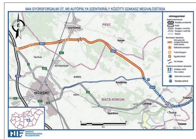
Az M44-es gyorsforgalmi út utolsó szakaszának nyomvonalja
